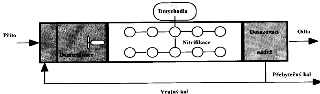
Obr. 1: Schematické znázornění aktivačního D-N systému
